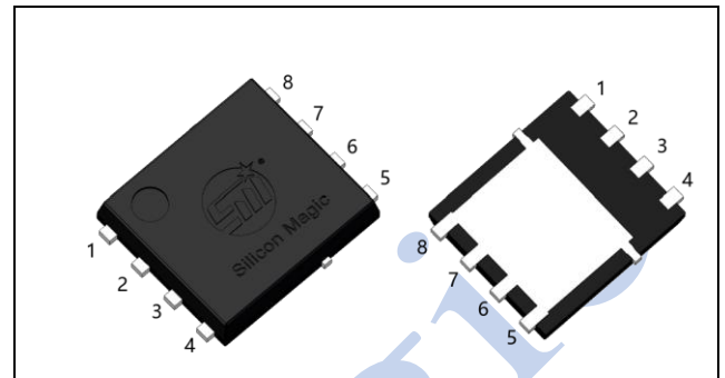
PDFN5X6-8L
