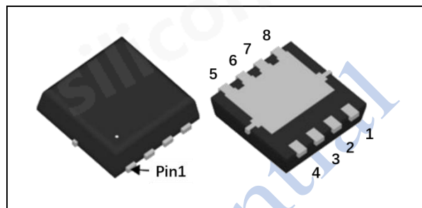
PDFN3.3*3.3-8L
